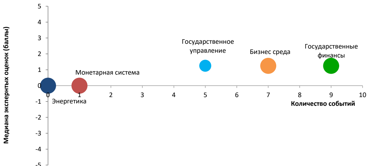
График 4. Значение отдельных компонентов Индекса и количество событий за период с 19 декабря 2016 по 8 января 2017г.
